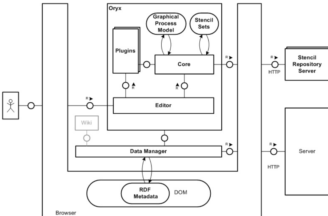
Abbildung 4.4: Architektur - Diagramm
